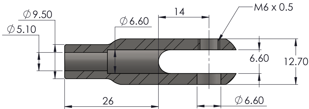
SECTION A-A SCALE 2 : 1.2
